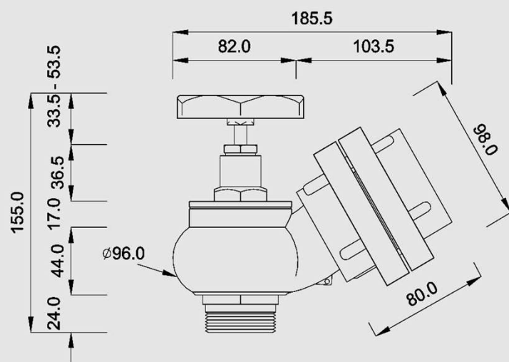
VISTA LATERAL
