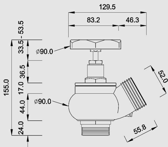
VISTA LATERAL
