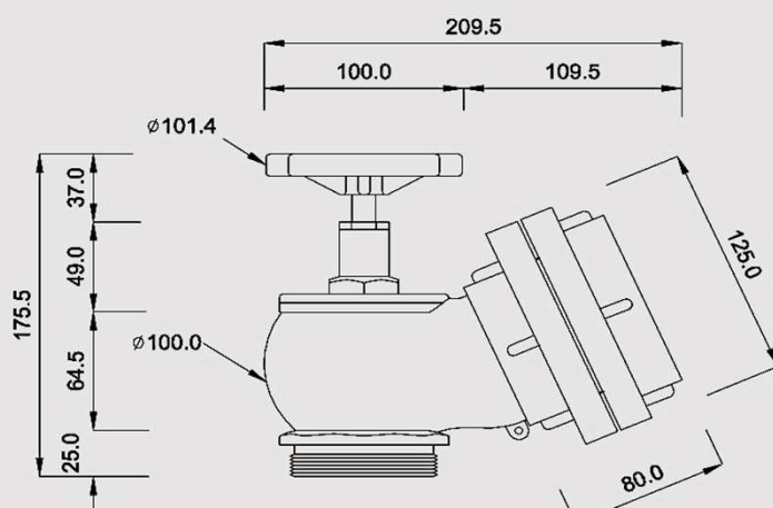
VISTA LATERAL
